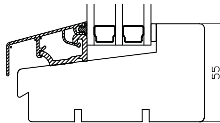
UNDERSTYCKE MED ALUMINIUMSKENA
