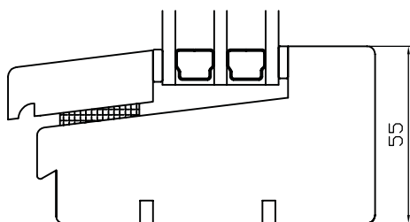
UNDERSTYCKE MED TRÄLIST
