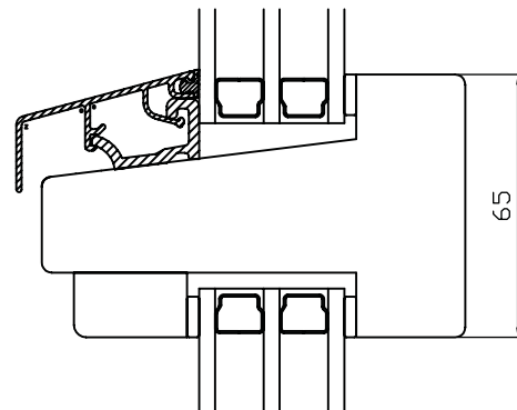
TVÄRPOST MED ALUMINIUMSKENA
