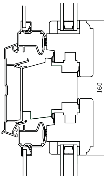
TVÄRPOST
