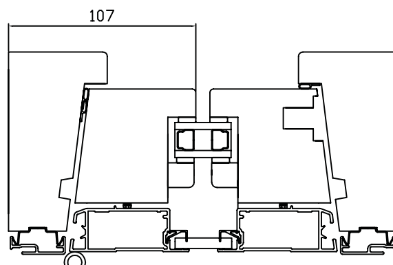
HORIZONTALSNITT
