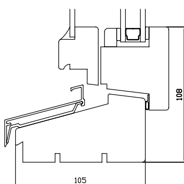
UNDERSTYCKE ALU-SKENA 105 KARM
