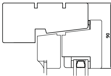
ÖVERSTYCKE 105 alt. 118 KARM
